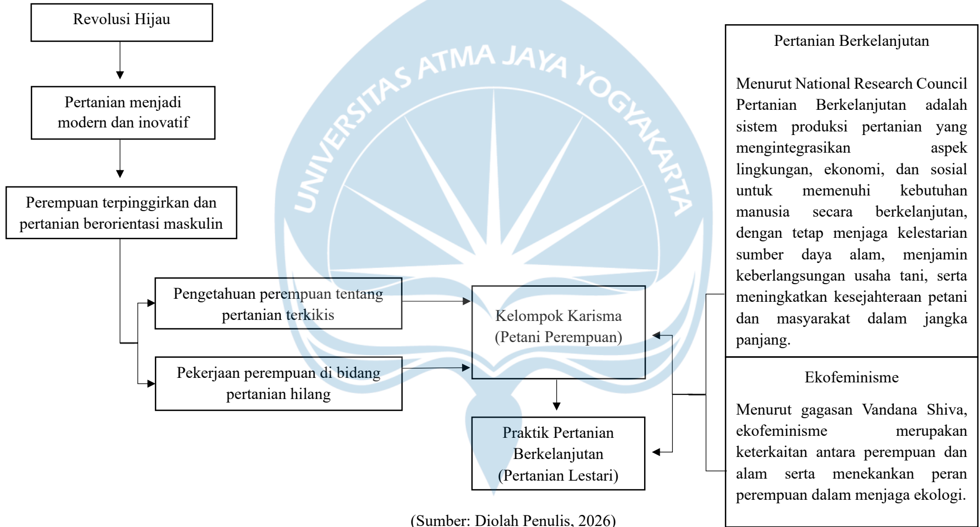
Gambar 1: Kerangka Berpikir
