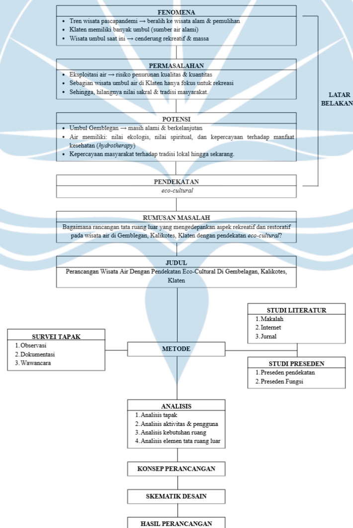
Gambar 1.4 Kerangka Berpikir
