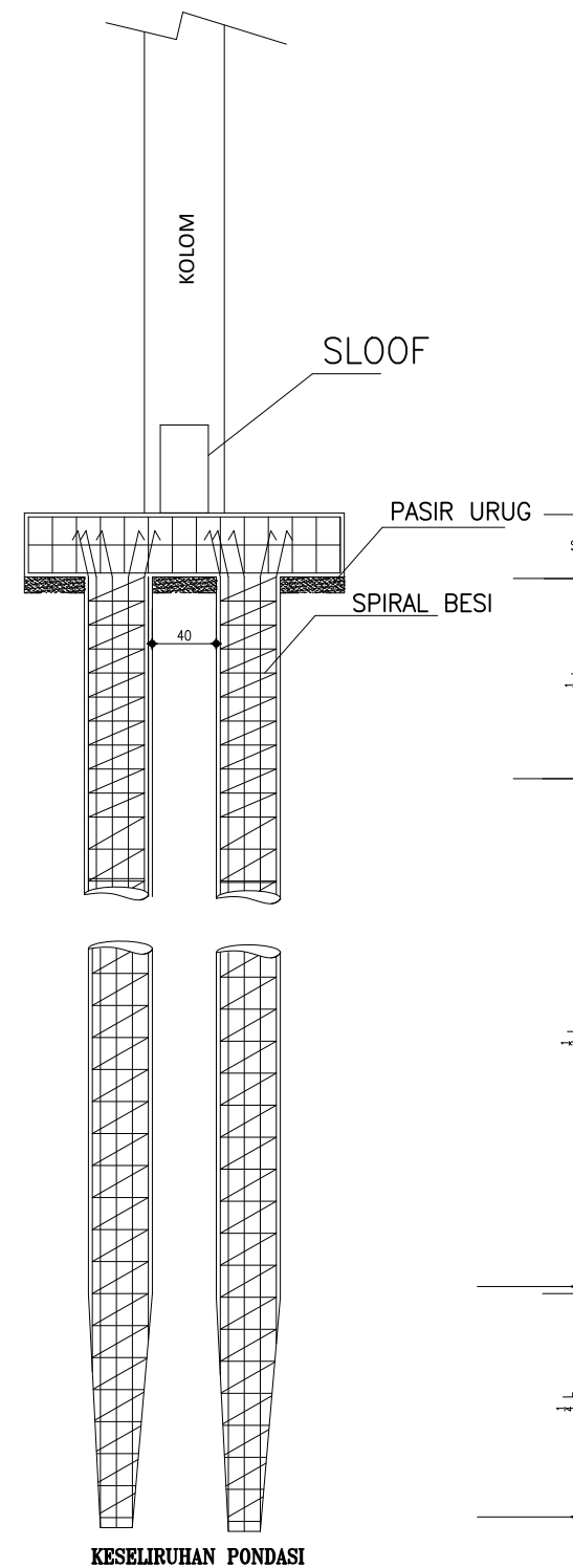
DETAIL PENEKANAN DESAIN SKALA 1 : 20
