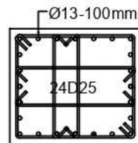
Potongan A-A SKALA 1: 25
