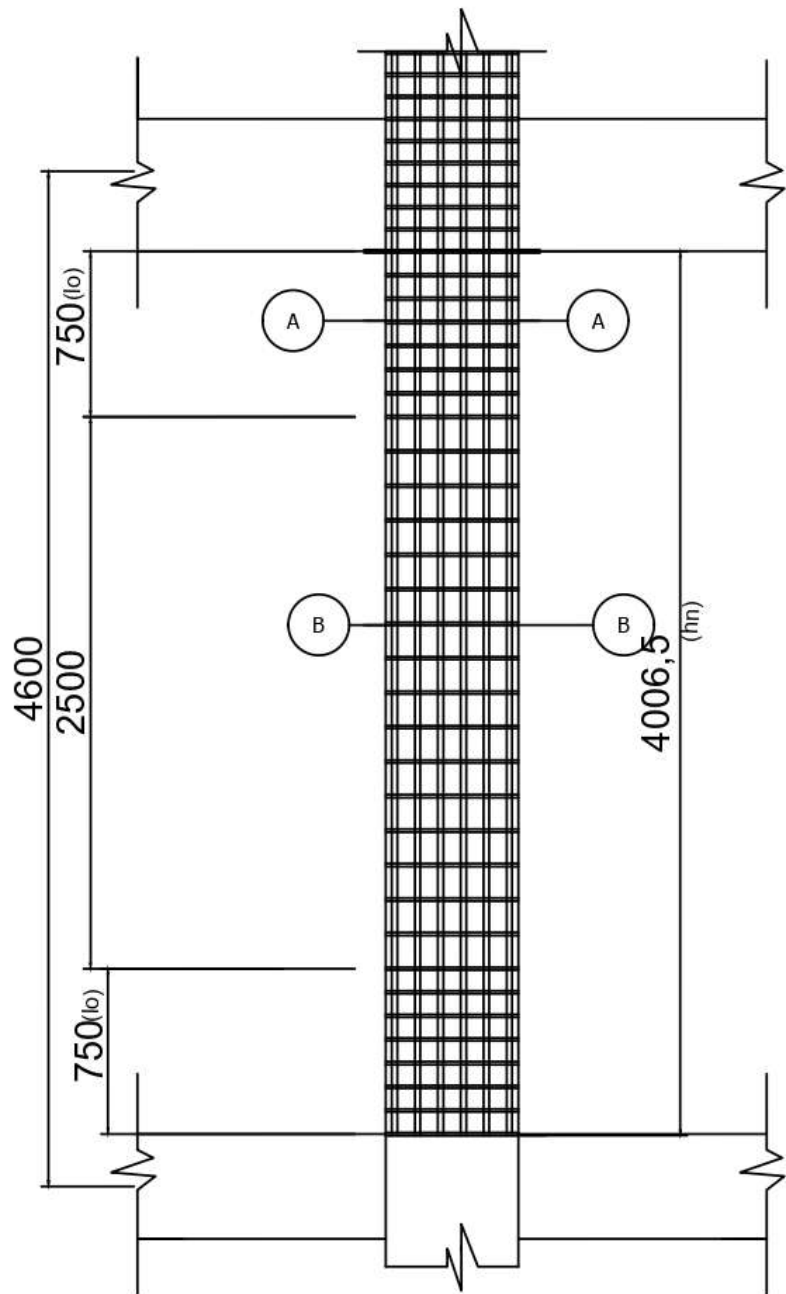
Detail Penulangan K3A SKALA 1: 25
