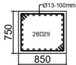
Potongan B-B SKALA 1: 25
