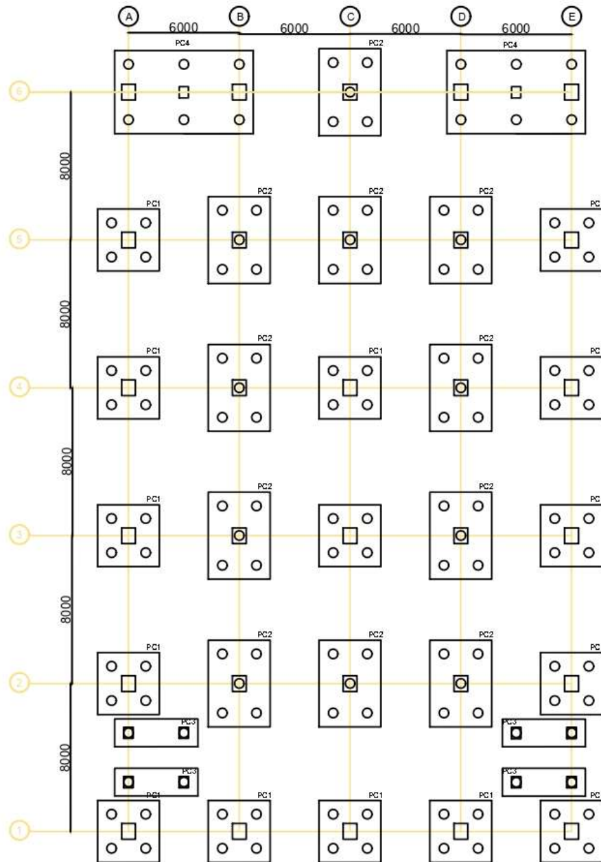
DENAH PONDASI 1:250
