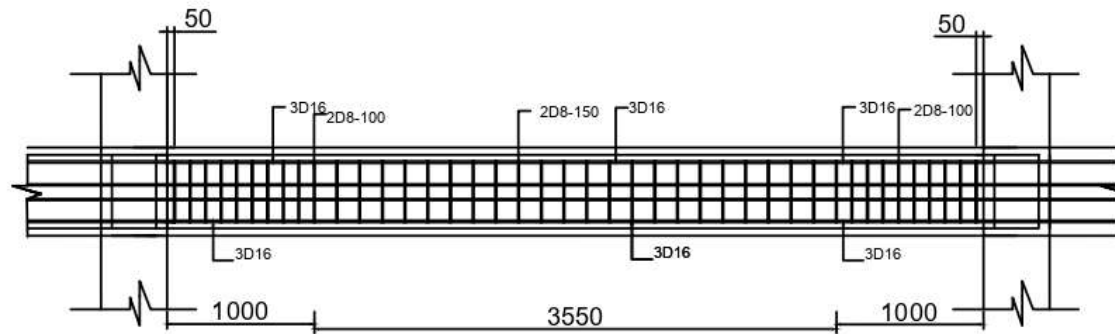
Detail Penulangan Ba 1 SKALA 1: 20
