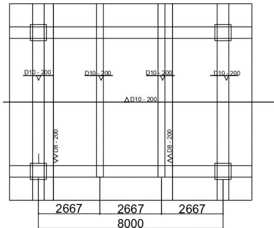
Detail Penulangan Pelat SKALA 1: 10
