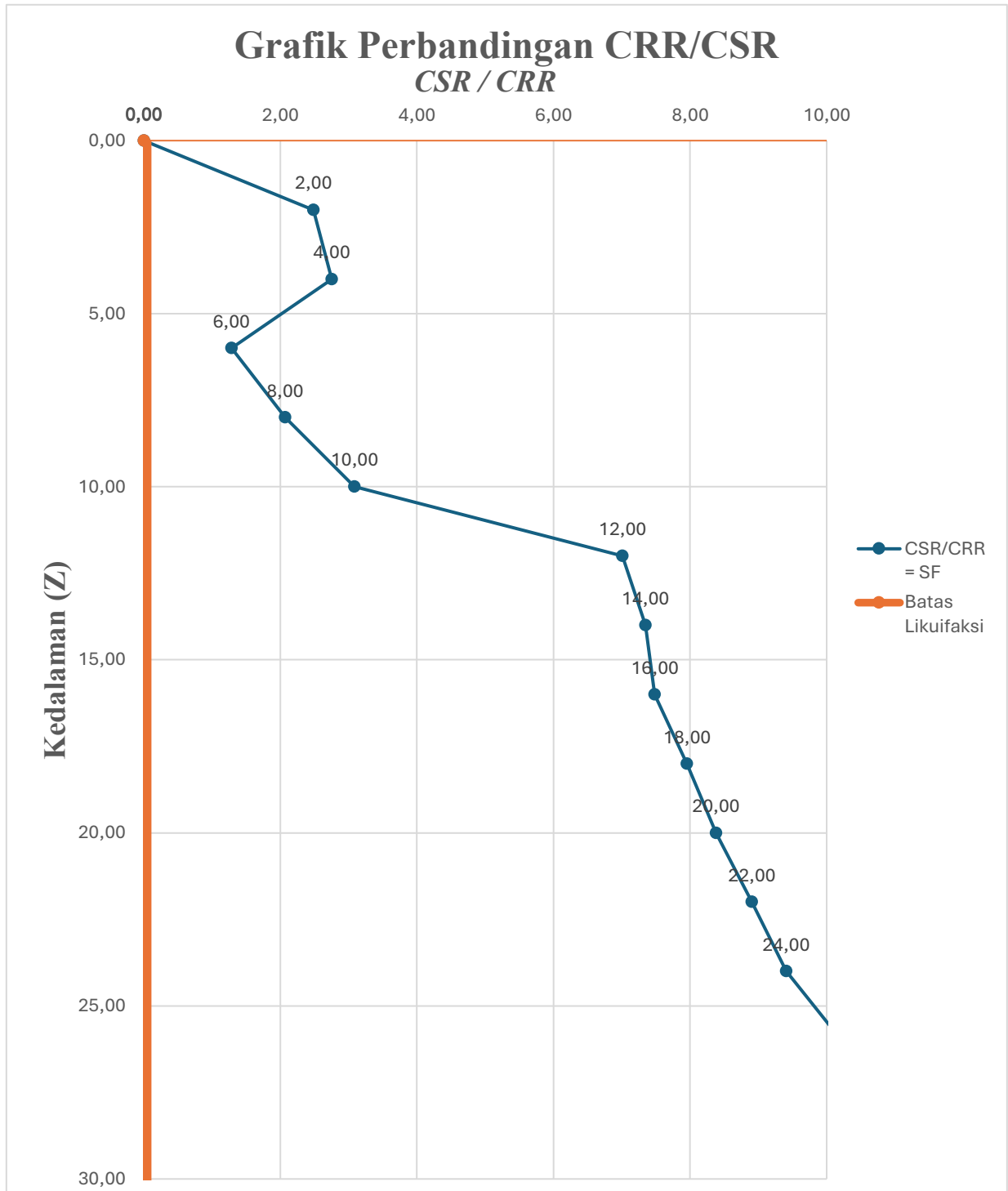
Gambar 3. 10 Grafik Perbandingan CRR dan CSR
