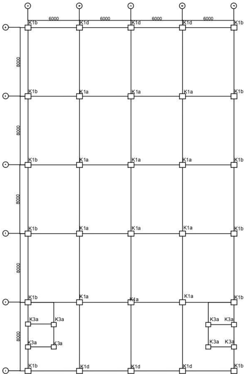
Denah Penulangan Kolom SKALA 1: 3
