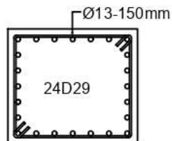
• Potongan B-B SKALA 1: 25
