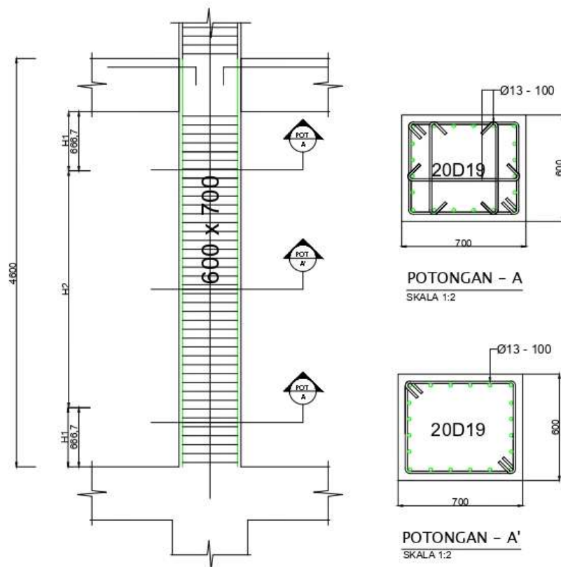
DETAIL KOLOM K2A
