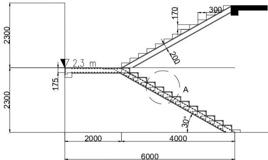
POT. A TANGGA 1
