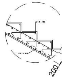
DETAIL ANAK TANGGA 1
