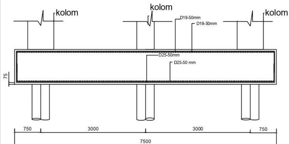
POTONGAN A SKALA 1: 4,5
