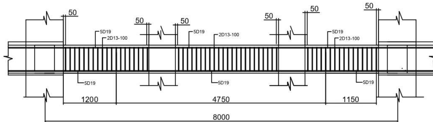
Detail Penulangan B1b SKALA 1: 20
