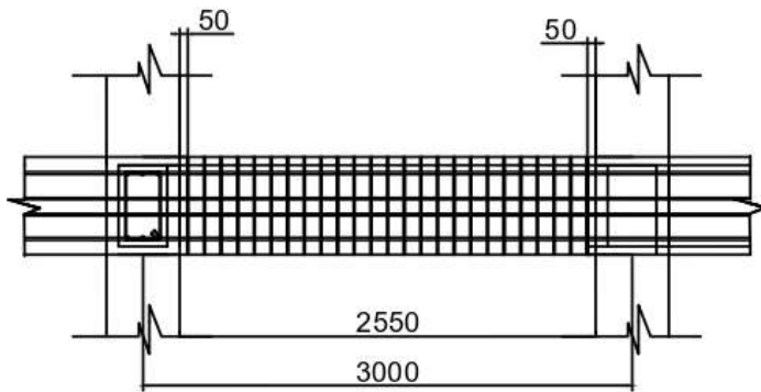
Detail Penulangan Ba 2 SKALA 1: 20
