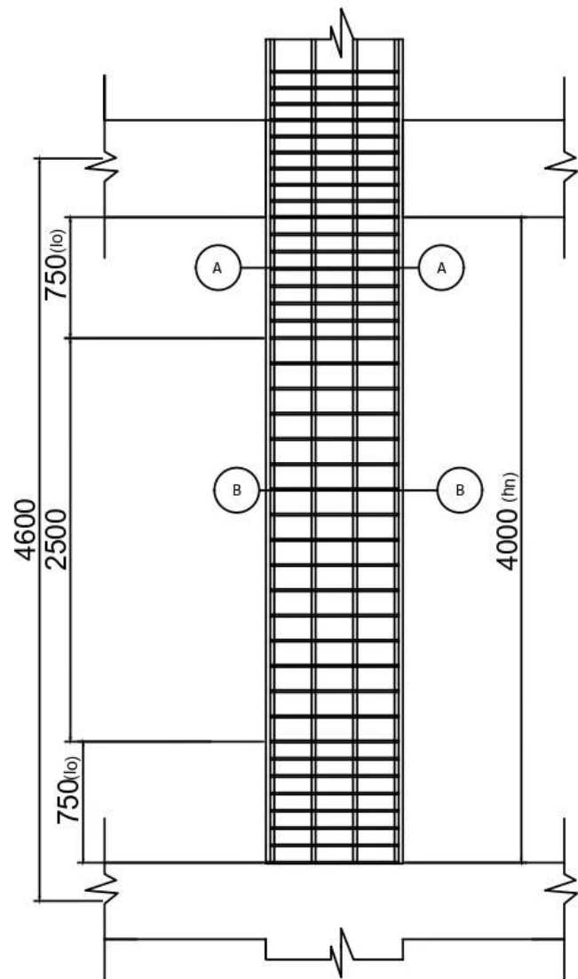
Detail Penulangan K1a SKALA 1: 25
