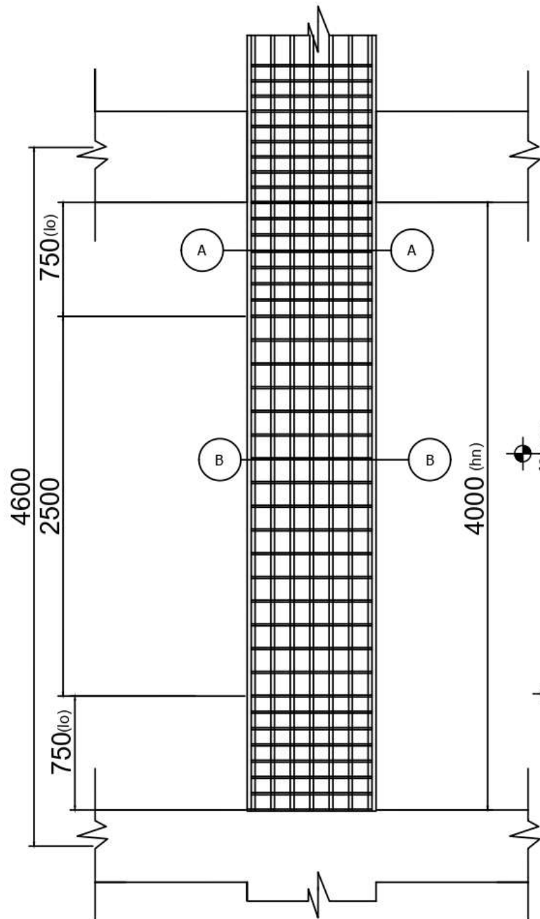
Detail Penulangan K1d SKALA 1: 25
