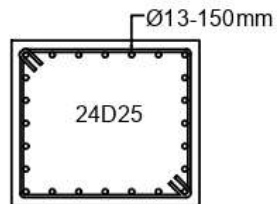
Potongan B-B SKALA 1: 25
