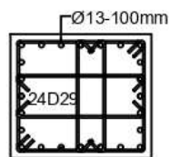
• Potongan A-A SKALA 1: 25
