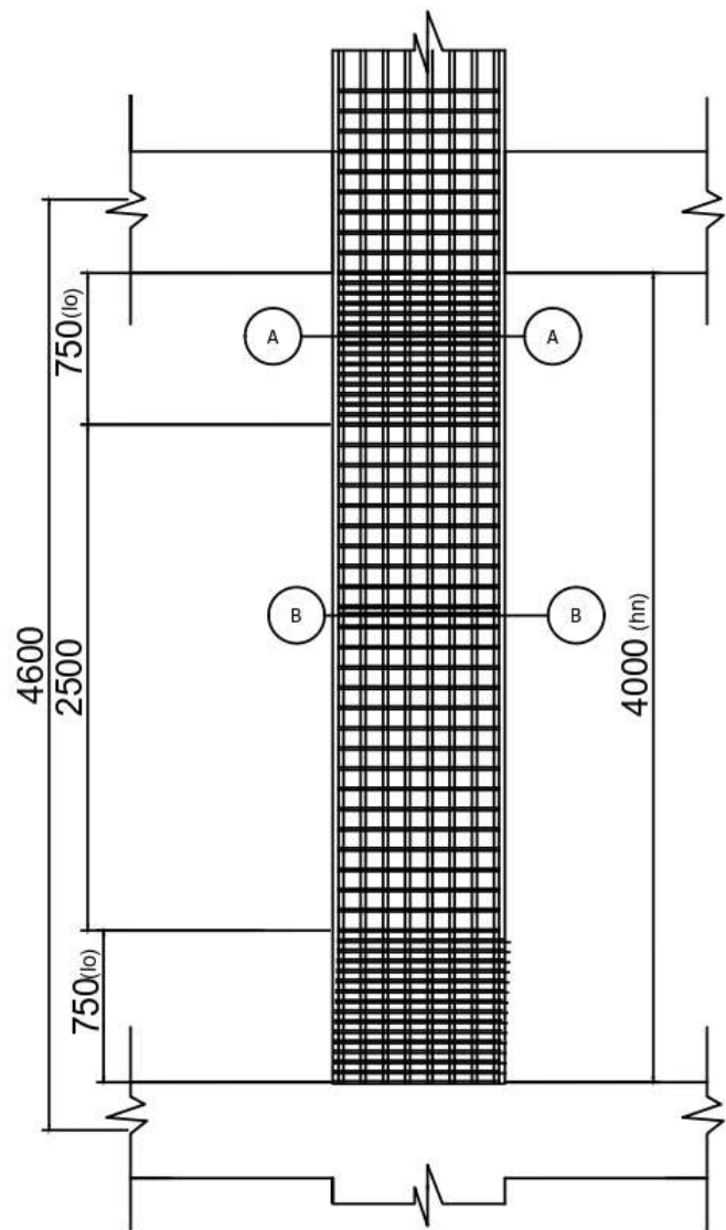
Detail Penulangan K1b SKALA 1: 25
