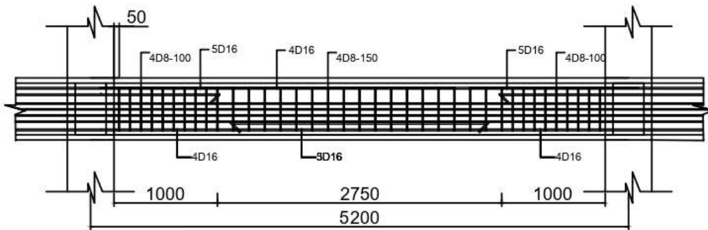
Detail Penulangan Ba 3 SKALA 1: 20
