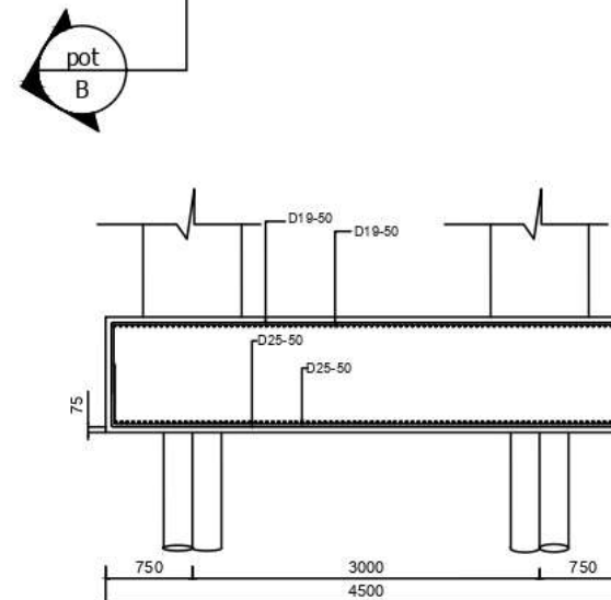
POTONGAN B SKALA 1: 4
