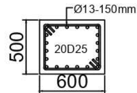
Potongan B-B SKALA 1: 25
