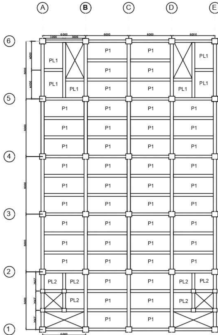
DENAH PENULANGAN PELAT LANTAI SKALA 1: 20
