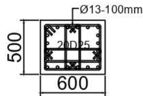
Potongan A-A SKALA 1: 25
