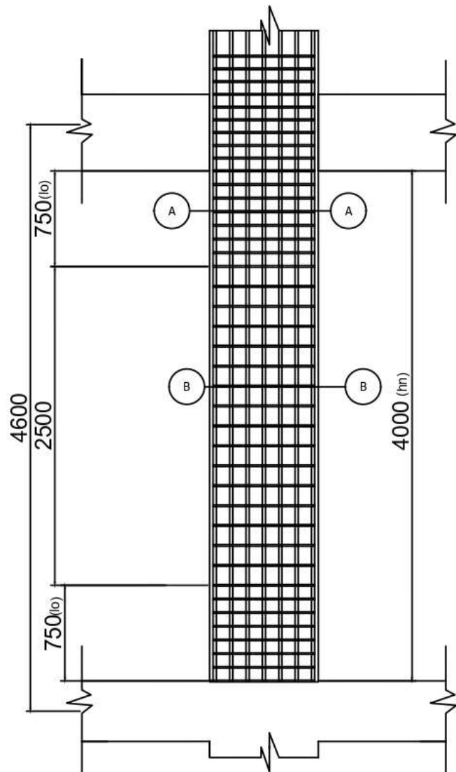
• Detail Penulangan K1c SKALA 1: 25
