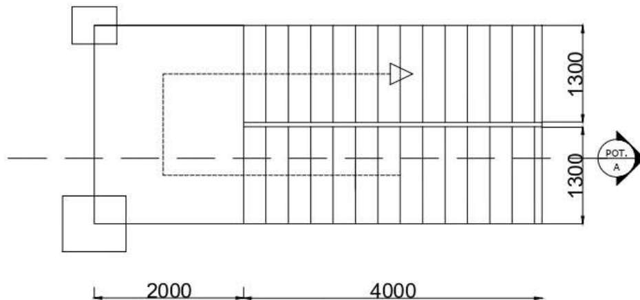
TAMPAK ATAS TANGGA 1
