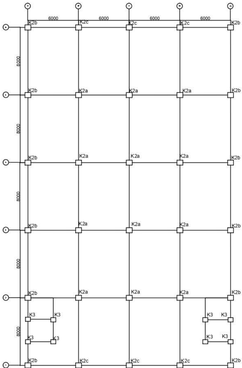
Denah Penulangan Kolom SKALA 1: 3
