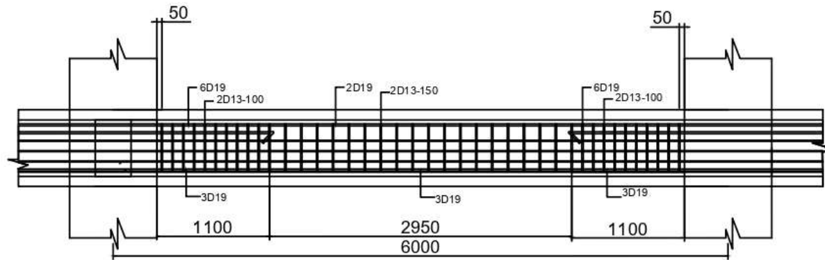
Detail Penulangan B2a SKALA 1: 20
