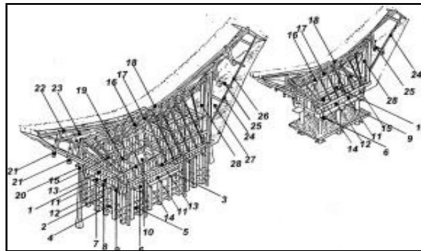
Gambar 2. 7 Konstruksi Togkonan dan Alang Sumber : (L. T. Tangdilintin, 1978)
