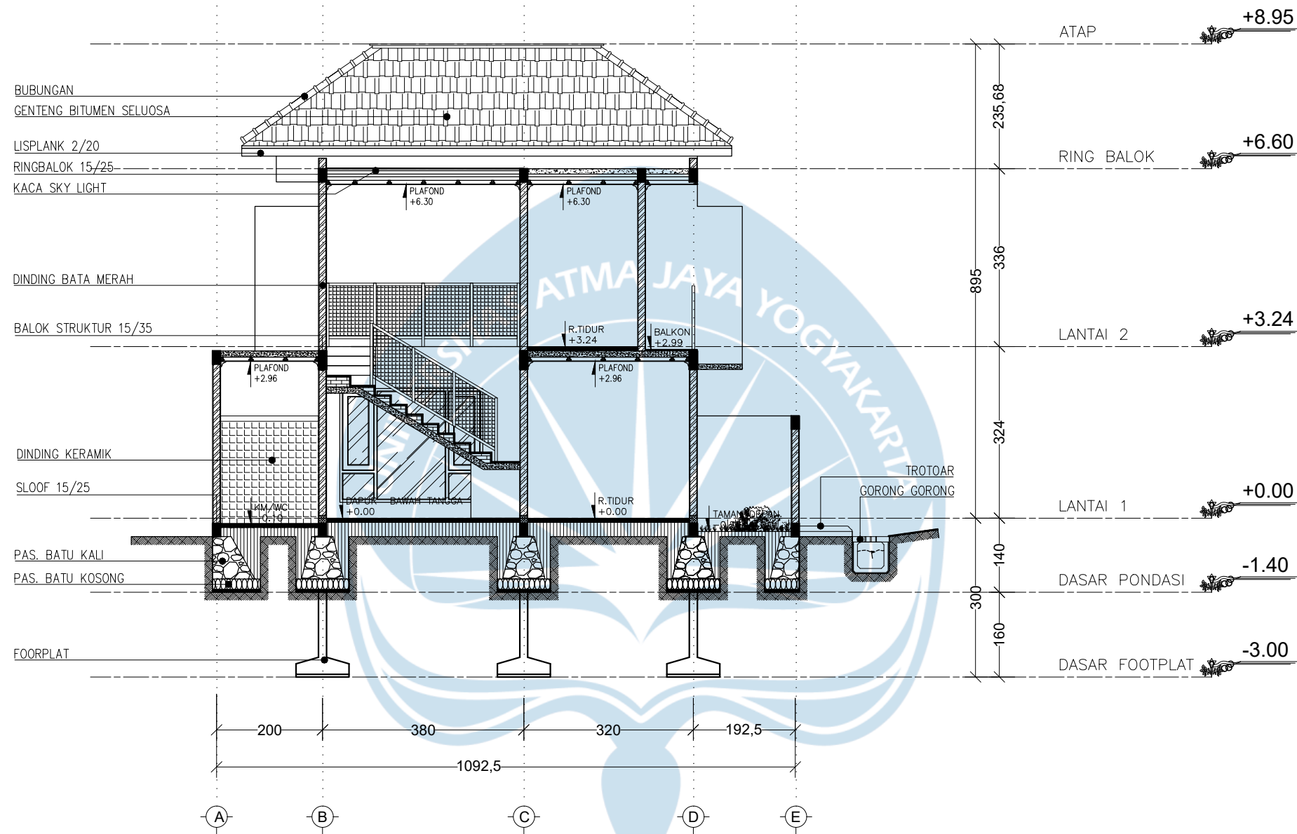
POTONGAN A-A B.TIPE 90 Skala 1: 100
