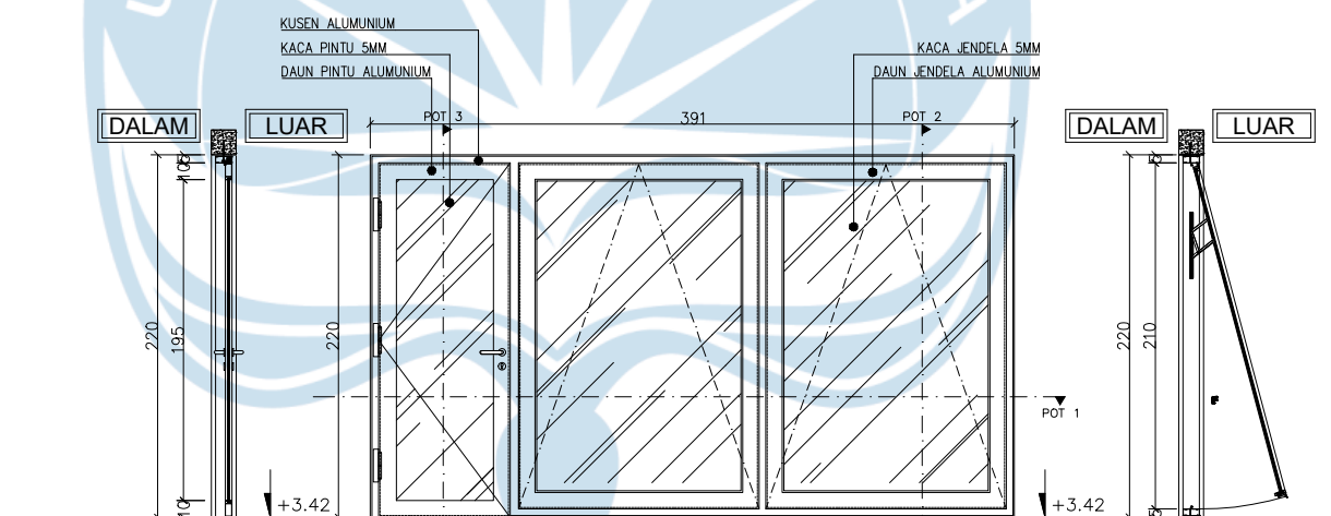
POTONGAN 3
