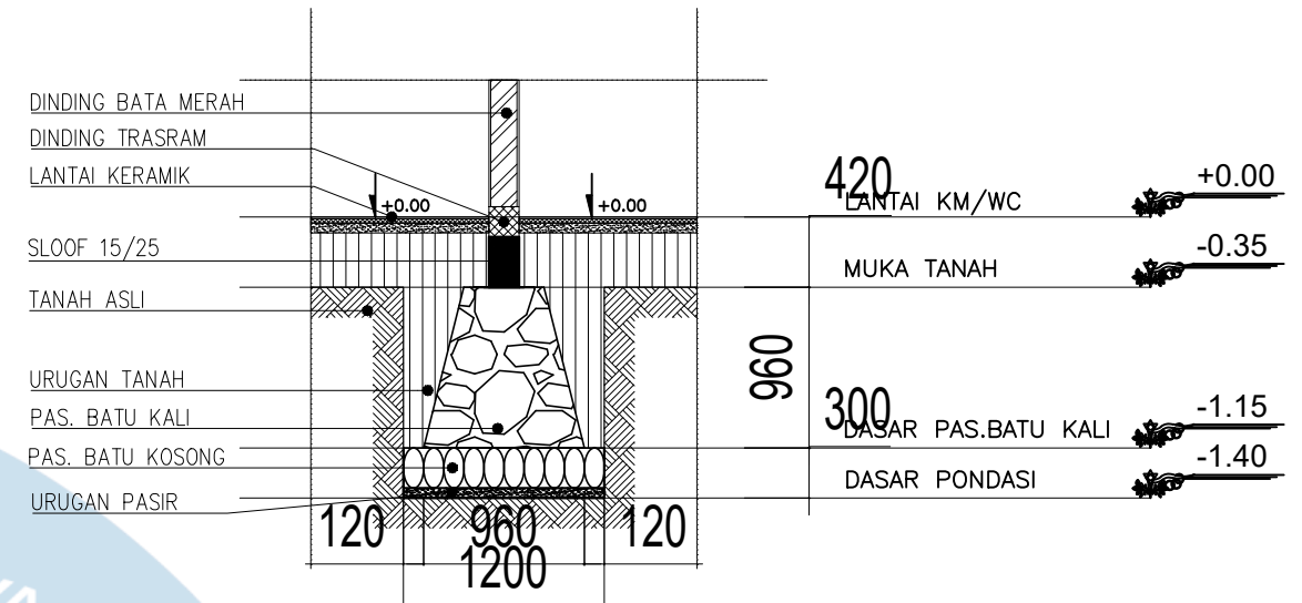
POTONGAN PONDASI A-A Skala 1: 50
