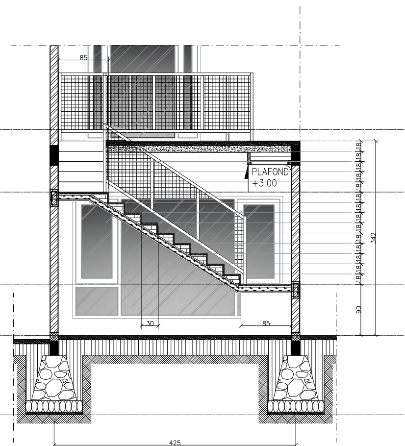
POTONGAN TANGGA A-A Skala 1: 30
