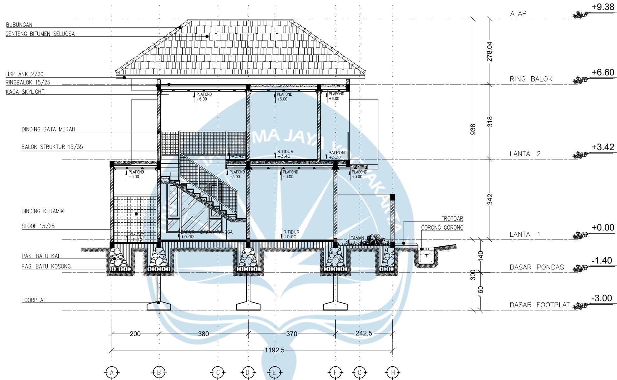
POTONGAN A-A TIPE 120 Skala 1: 100
