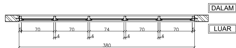
POTONGAN 1
