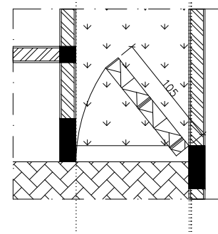
DETAIL PINTU ROOSTER Skala 1: 50
