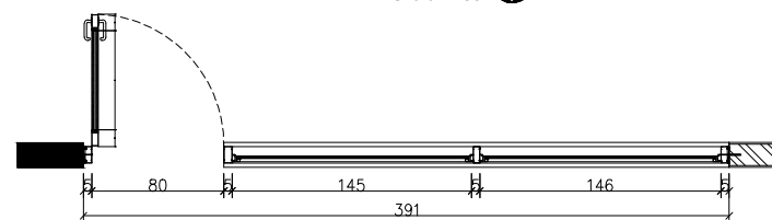
POTONGAN 1
