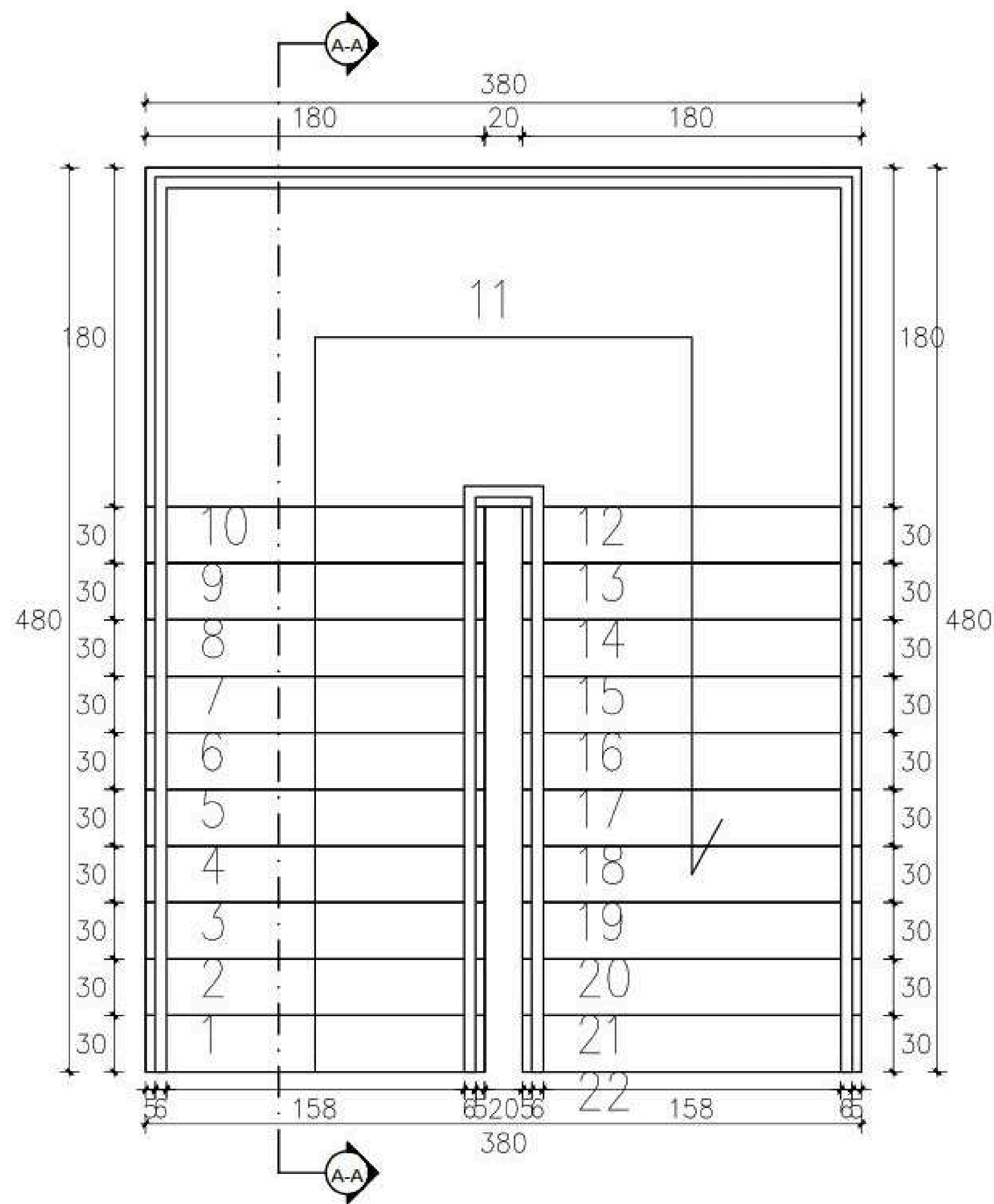
DETAIL TANGGA SCALE 1:50
