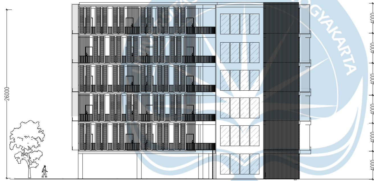
TAMPAK UTARA MASSA B SCALE 1 : 100
