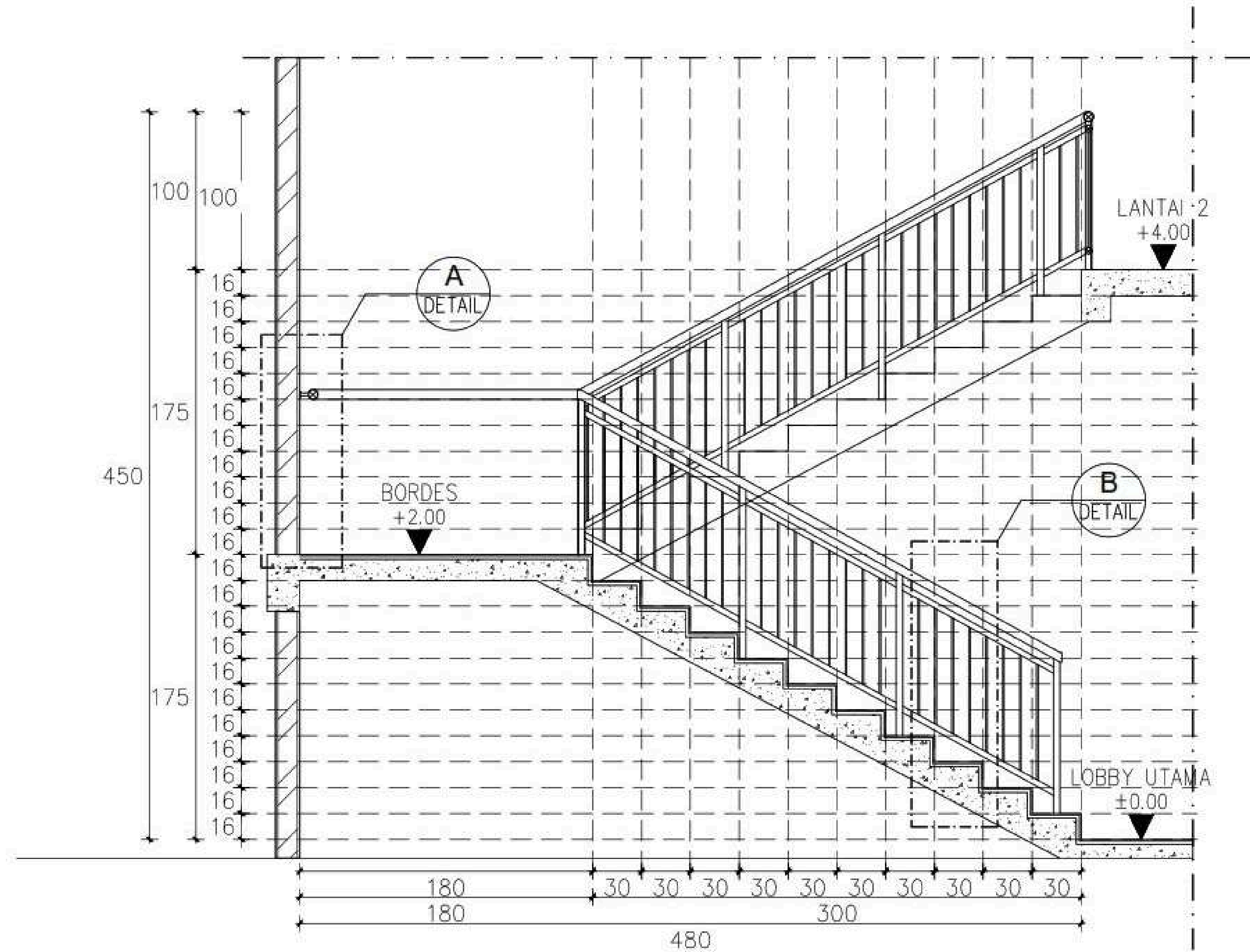
DETAIL A-A TANGGA SCALE 1:50
