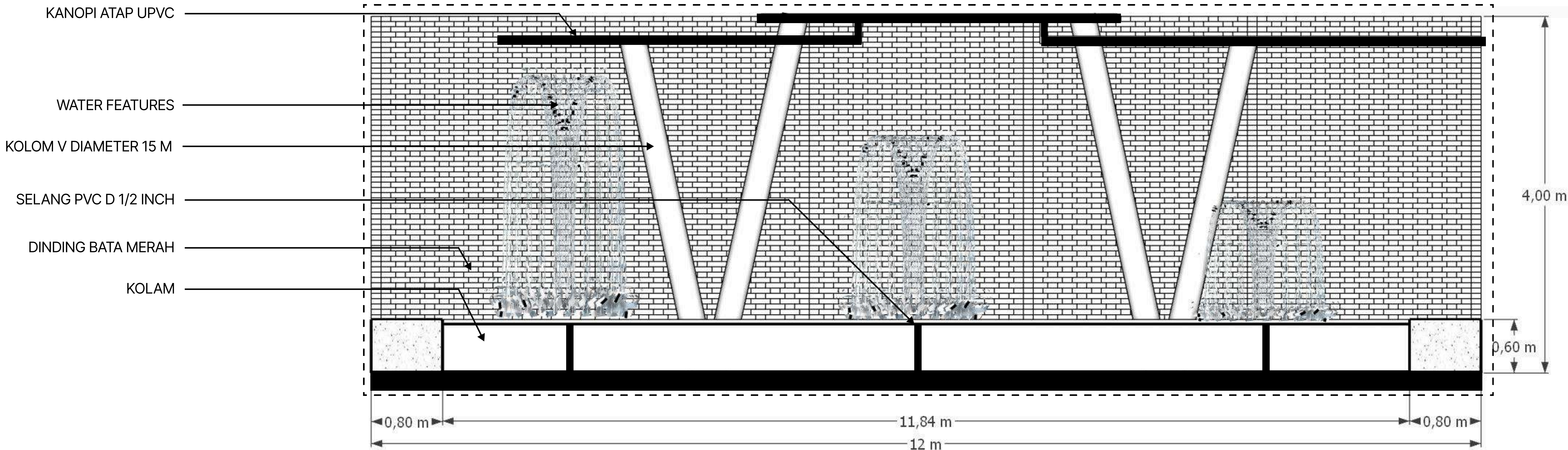
POTONGAN A-A SCALE 1:50
