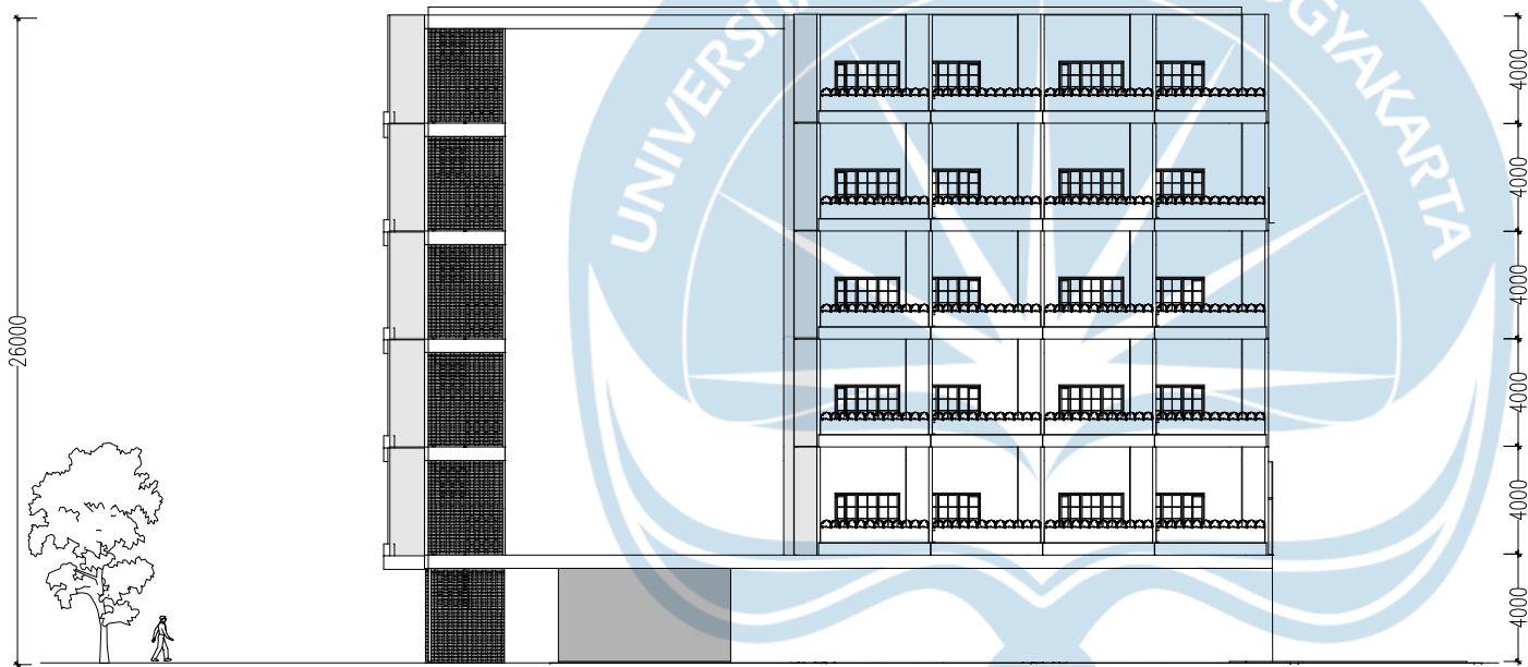
TAMPAK SELATAN MASSA B SCALE 1 : 100
