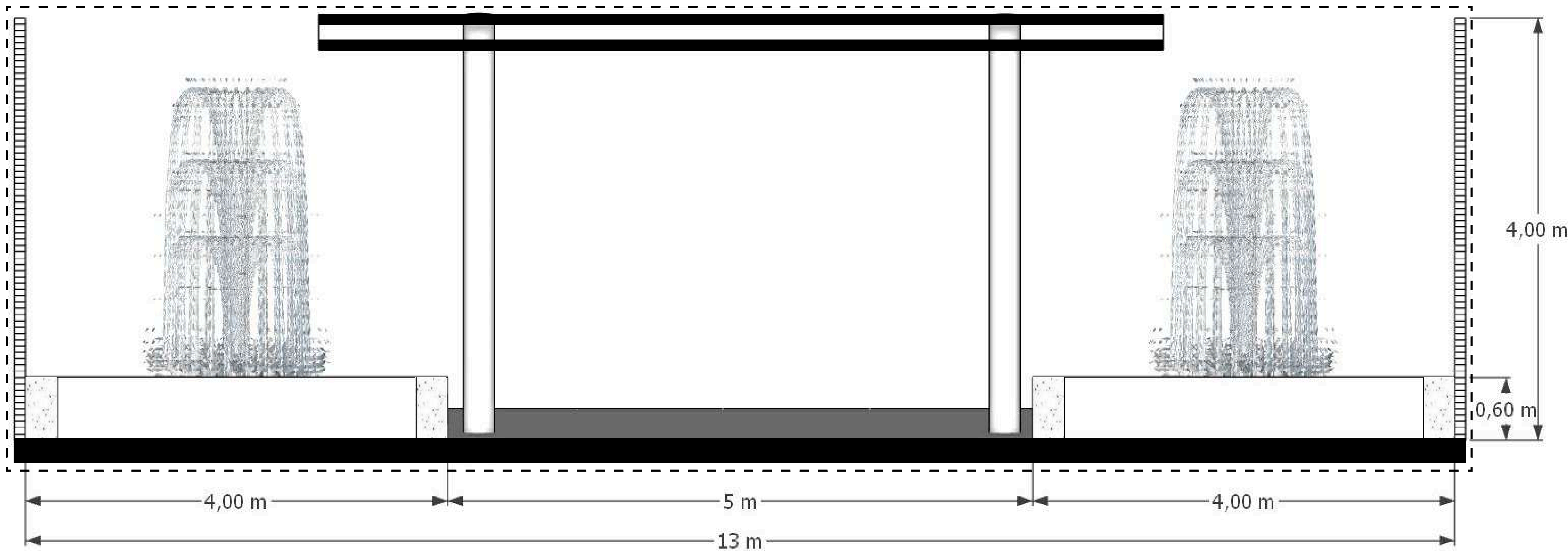
POTONGAN B-B SCALE 1:50
