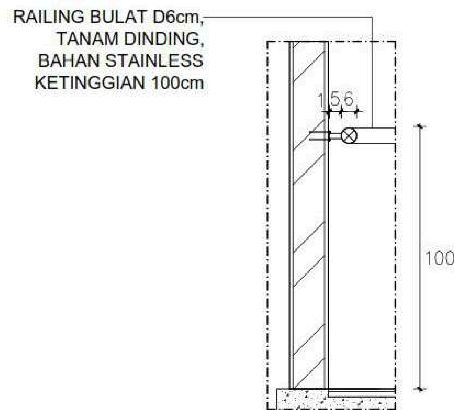
DETAIL A TANGGA SCALE 1:25
