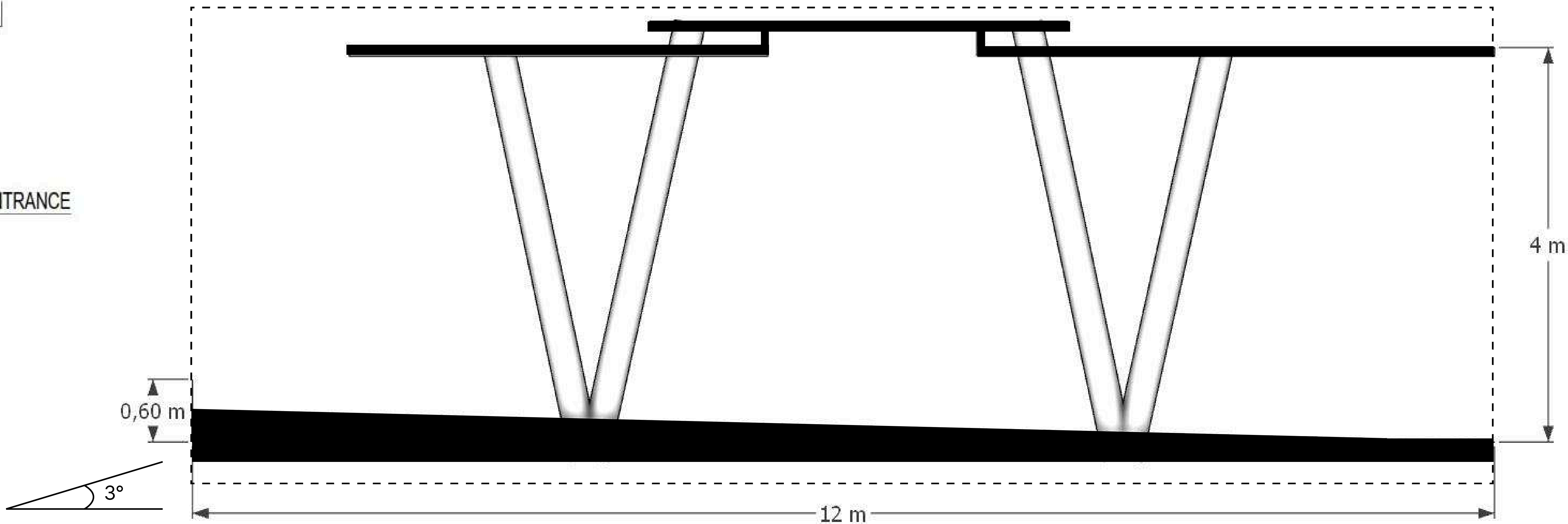
POTONGAN A-A SCALE 1:50
