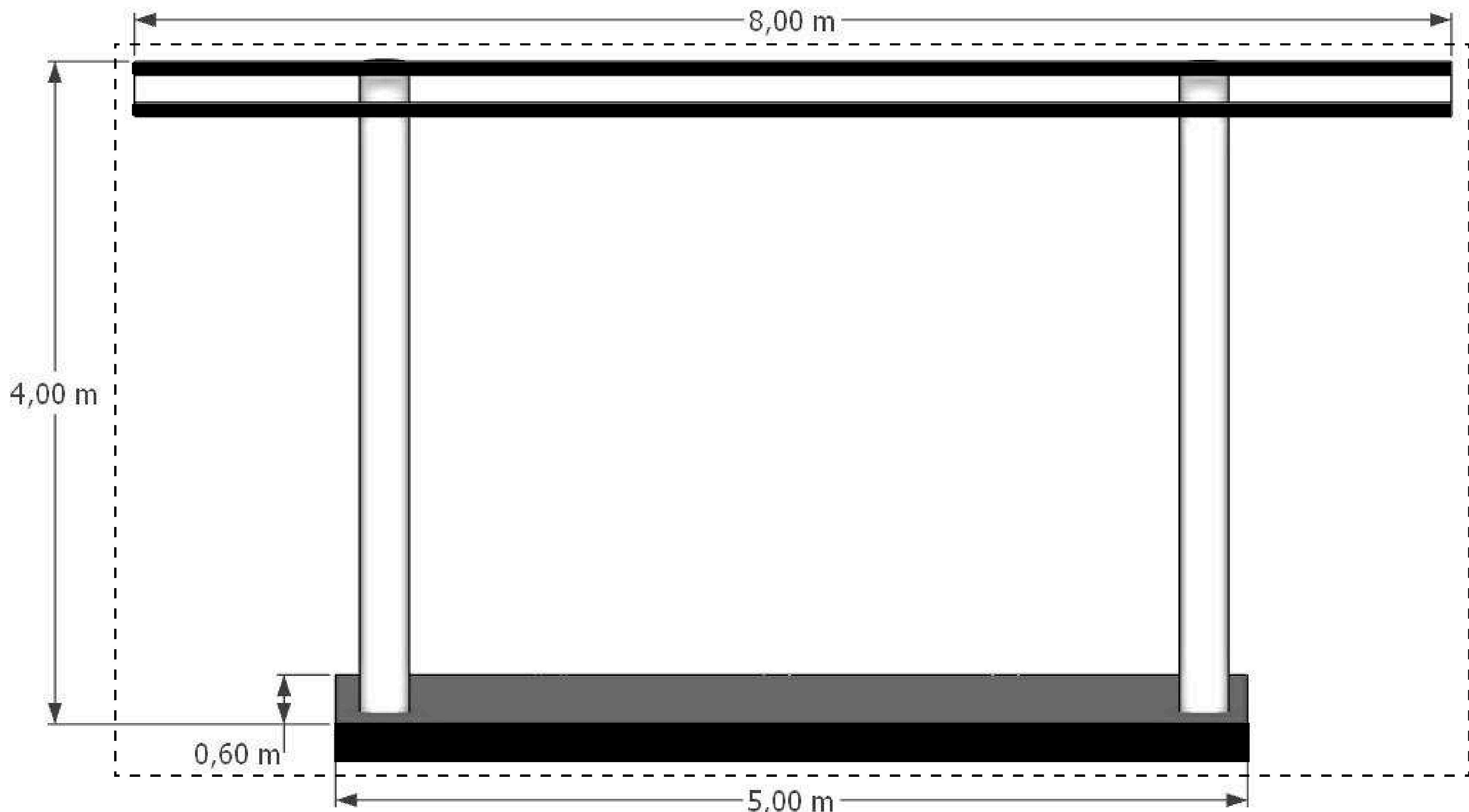
POTONGAN B-B SCALE 1:50
