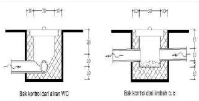
Rencana Air Kotor
