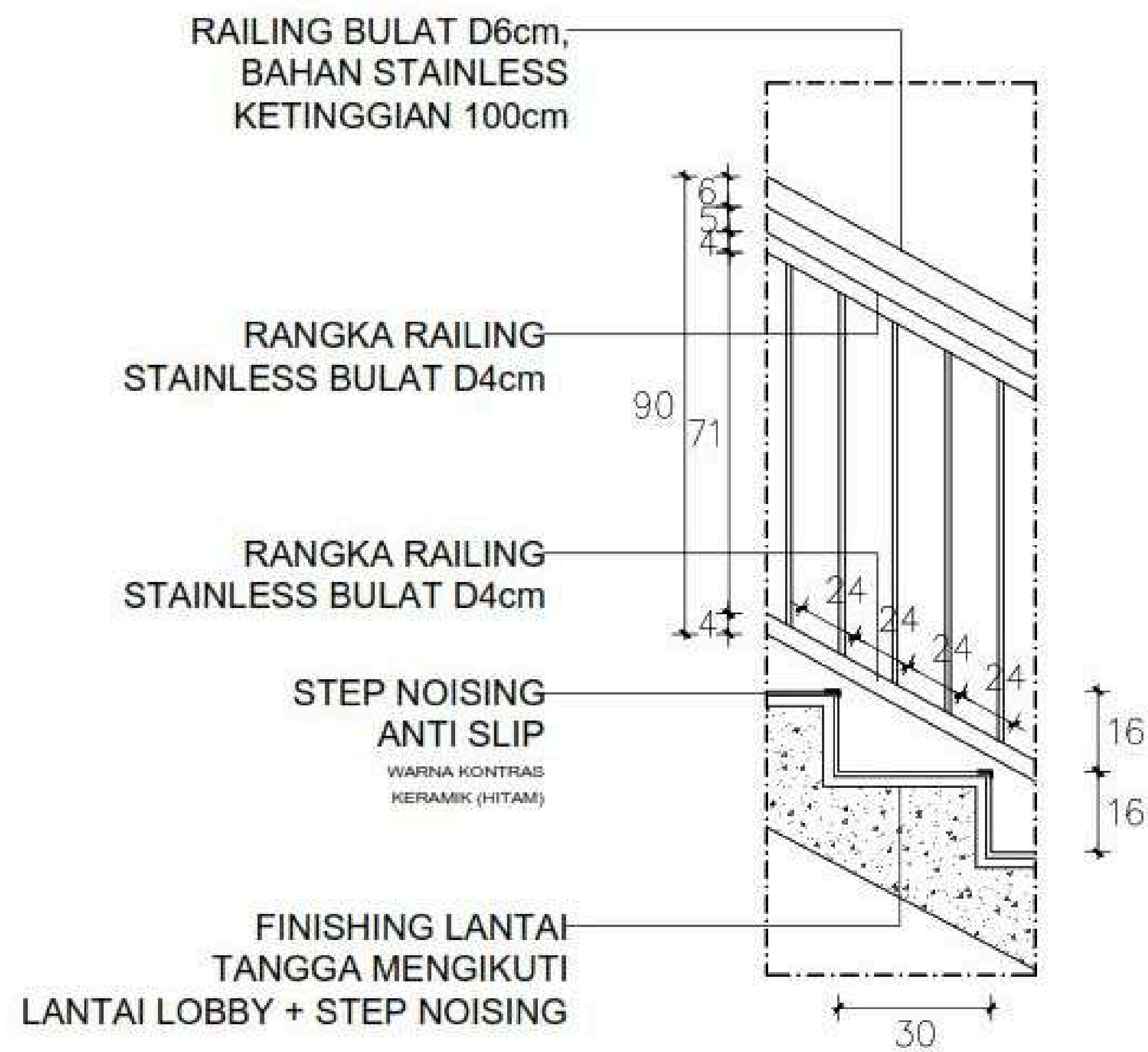
DETAIL B TANGGA SCALE 1:25
