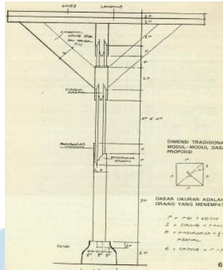
Gambar 2. 14 Struktur Kolom Puri Anom
