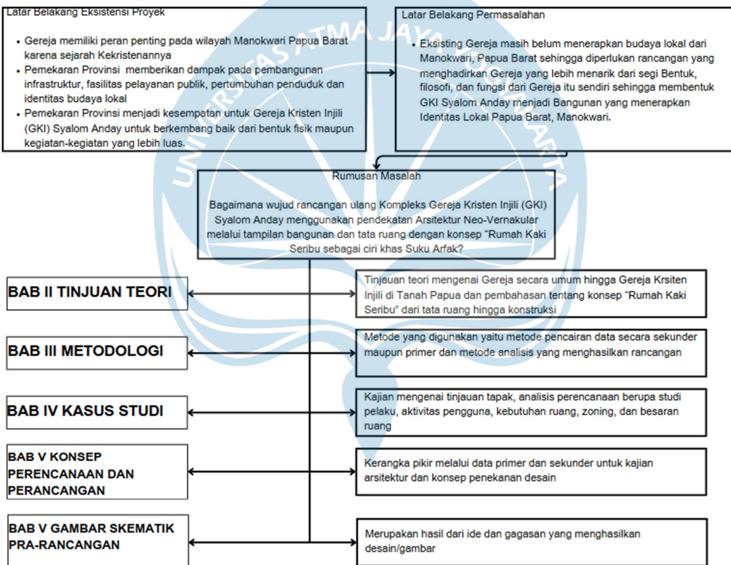
Gambar 1. 3 Kerangka Berpikir
