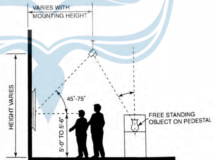
Gambar 2.11: Teknik Pencahayaan Buatan pada Ruang Pameran Sumber: Time-Saver Standards , 2001
