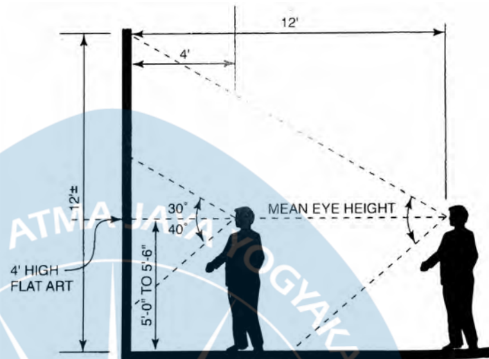
Gambar 2.10: Jarak dan Sudut Penglihatan pada Ruang Pameran Sumber: Time-Saver Standards , 2001
