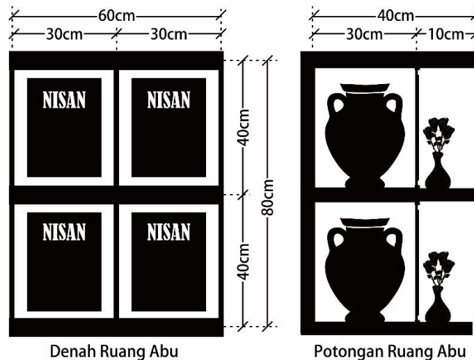
Gambar 2. 7 Denah dan Potongan Kolumbarium Pohsarang Sumber : Penulis 2020
