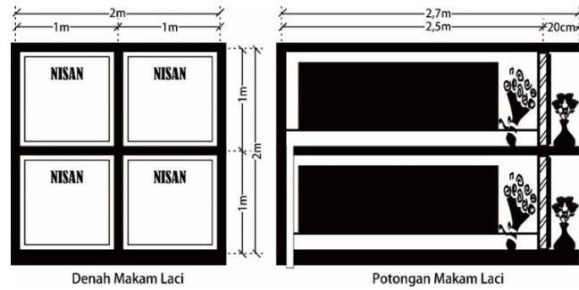
Gambar 2. 10 Denah dan Potongan Makam Laci Pohsarang
