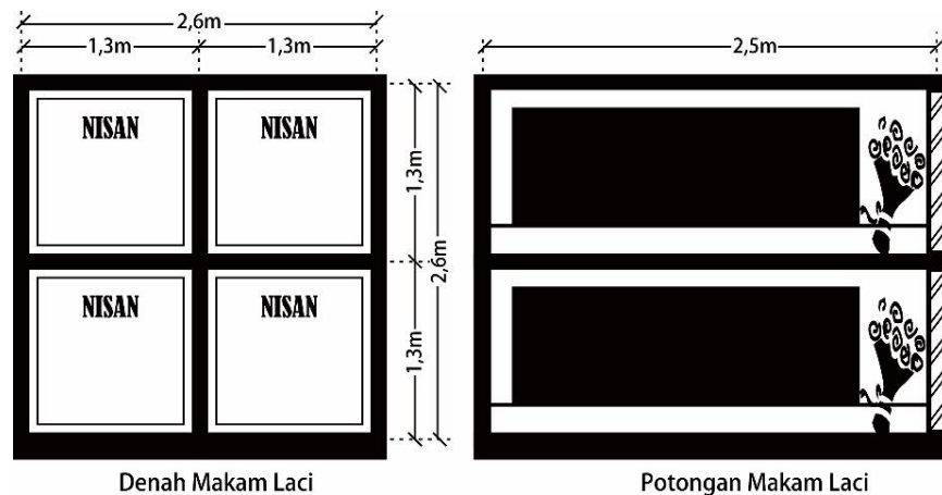
Gambar 2. 13 Denah dan Potongan Makam Laci Kerkof
