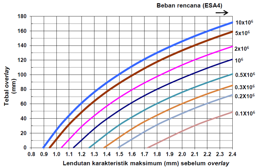
Gambar 3.2 Solusi Overlay berdasarkan Lendutan Balik Benkelman Beam
