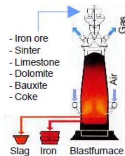
Gambar 2.1 Diagram proses produksi Iron Slag
