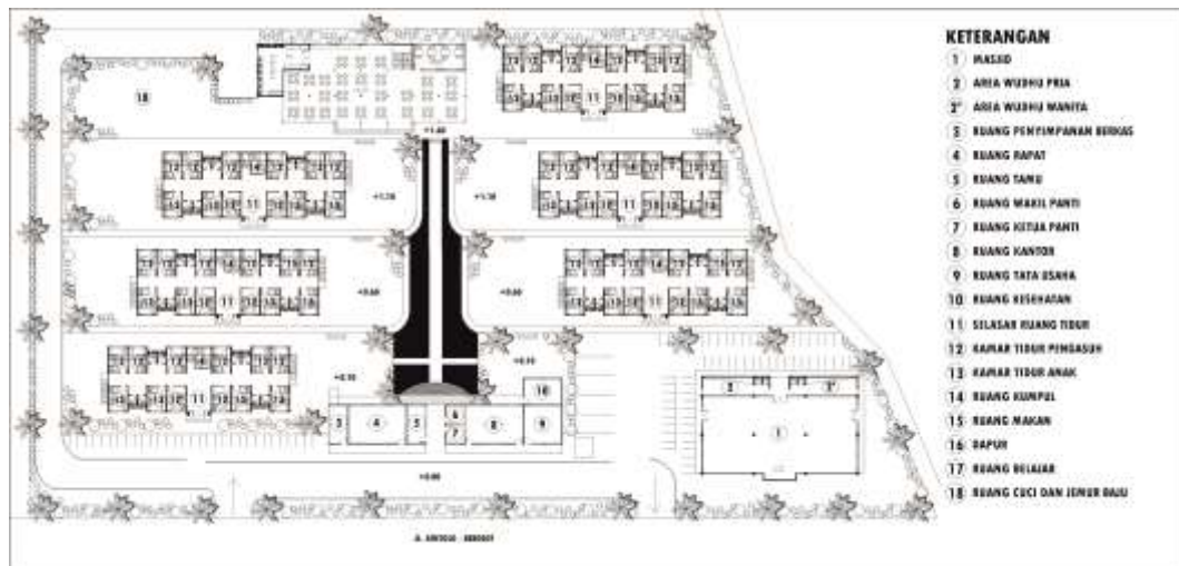
Gambar 7.4.2.1 Blok Plan
