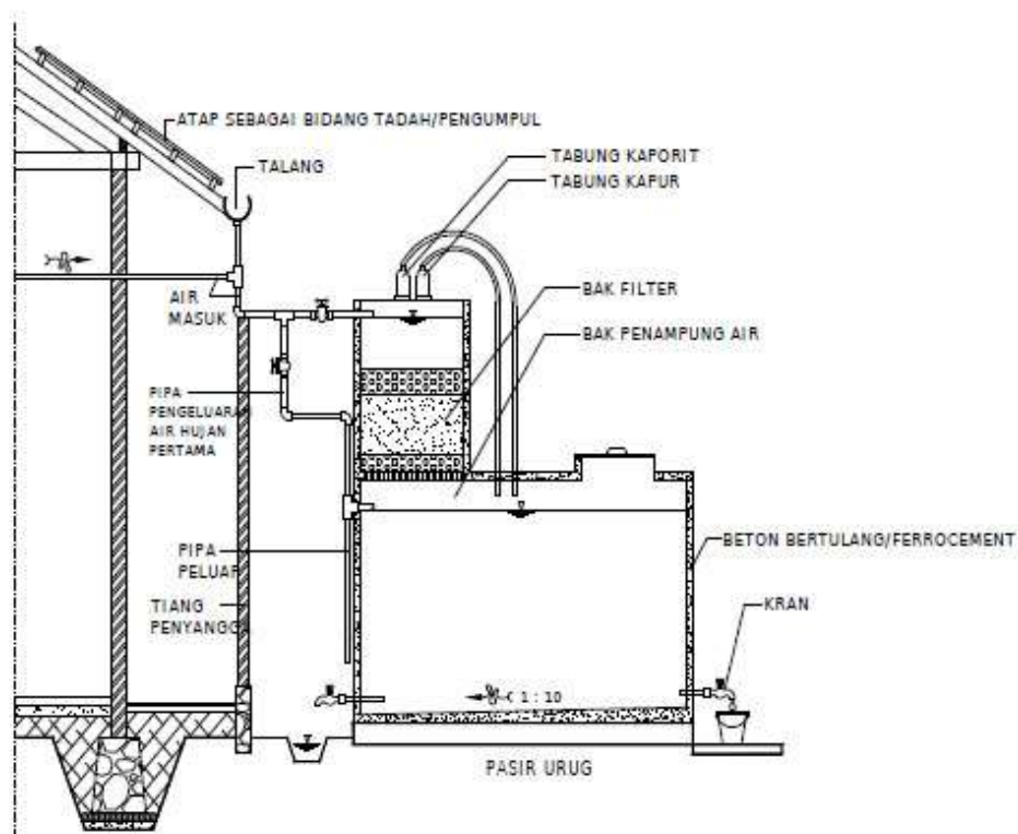
Gambar 7.6.2.1 Detail Penampungan Air Hujan
