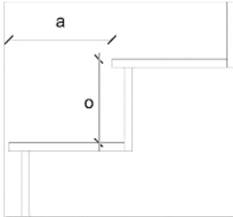
Gambar 7.4.3.1.5 Anak Tangga
