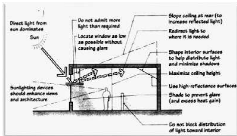
Gambar 7.7.1 Pencahayaan Alami
