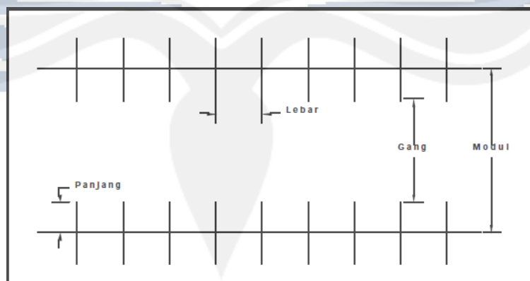
Gambar 3.4 Dimensi Jalur Gang untuk Pola Parkir sudut 90°
