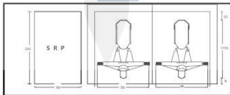
Gambar 3.3. Satuan Ruang Parkir untuk Sepeda Motor (dalam cm)
