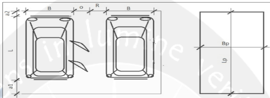
Gambar 3.1 Satuan Ruang Parkir untuk Mobil Penumpang (dalam cm)
