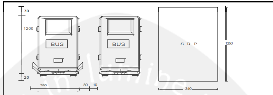
Gambar 3.2. Satuan Ruang Parkir untuk Bus / Truck (dalam cm)
